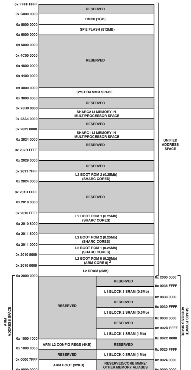
Figure 5. ADSP-SC57x/ADSP-2157x Memory Map
