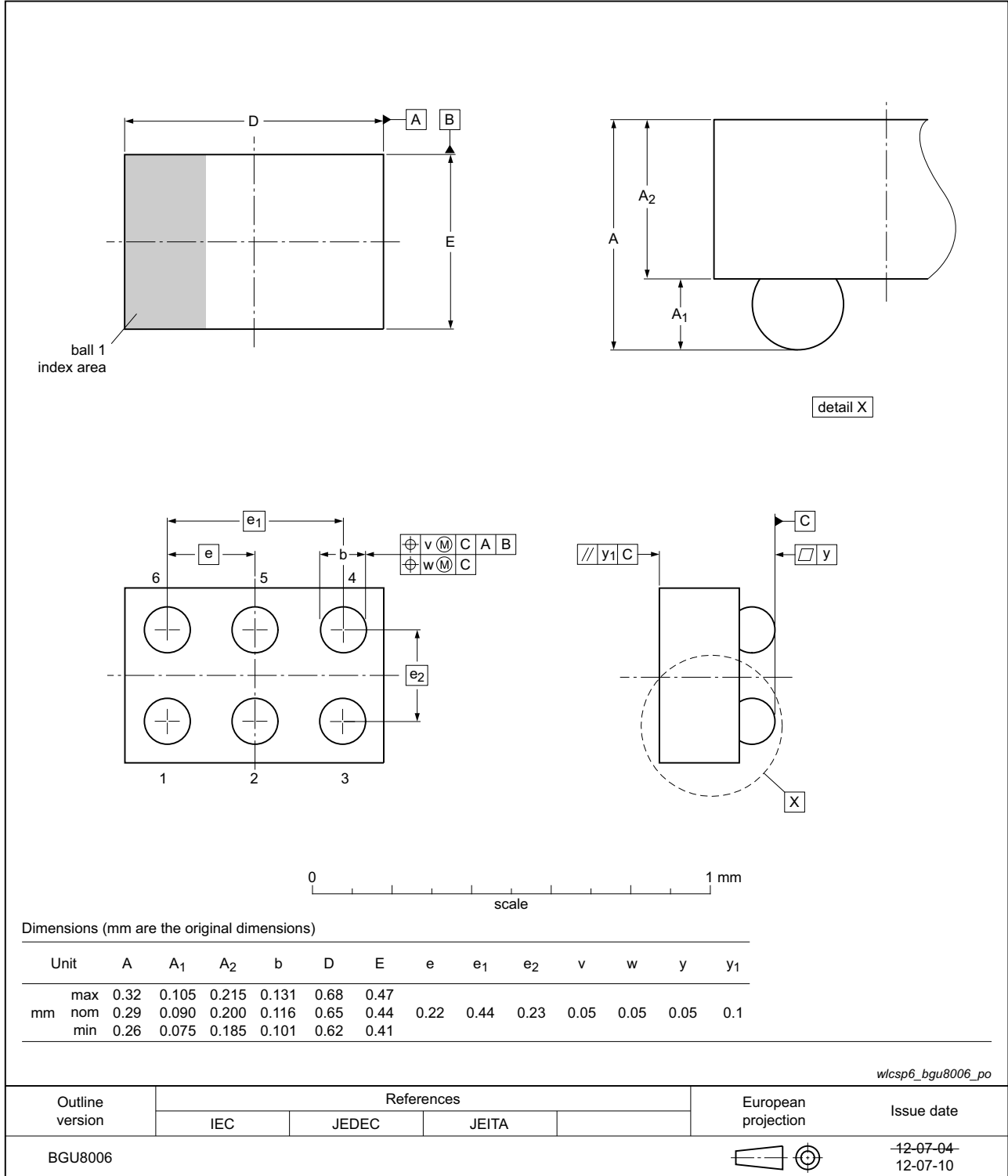
Fig 33. Package outline BGU8006 (WLCSP6)
